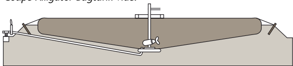
Coupe Alligator Bagtank rempli.
