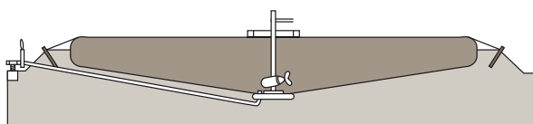
Sezione del prodotto Alligator Bagtank pieno.
