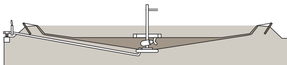
Prierez Alligator Bagtank (prázdny).
